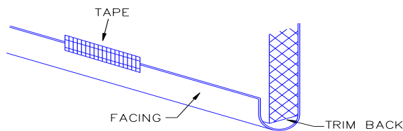
IL. 5.5 DOBLADO Y ENCINTADO DE REVESTIMIENTO
