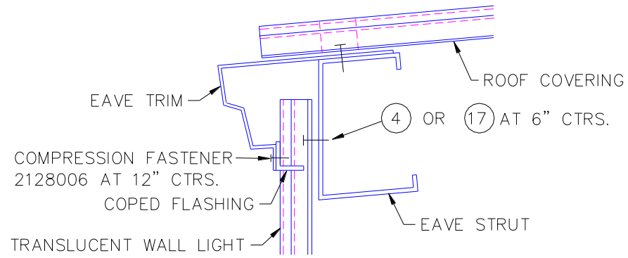
IL. 6.40 FIJACIÓN DE MOLDURA A PANEL TRANSLÚCIDO
