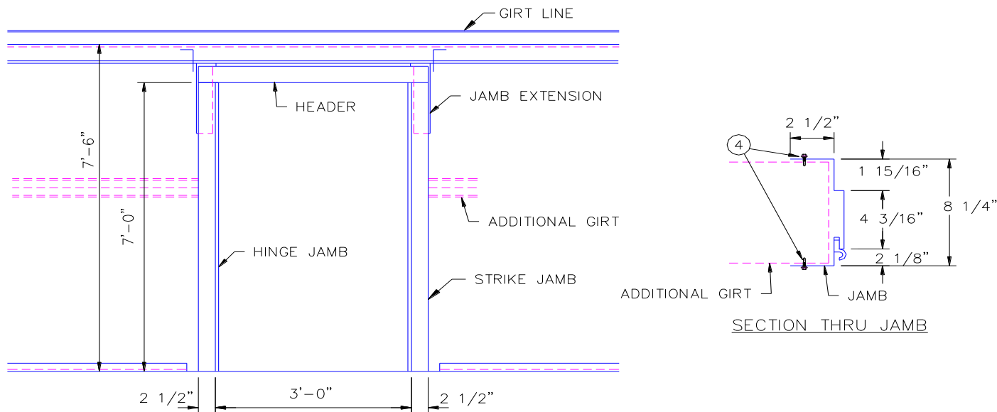
IL. 6.13 MARCO DE PUERTA DE ENSAMBLAJE EN CAMPO
