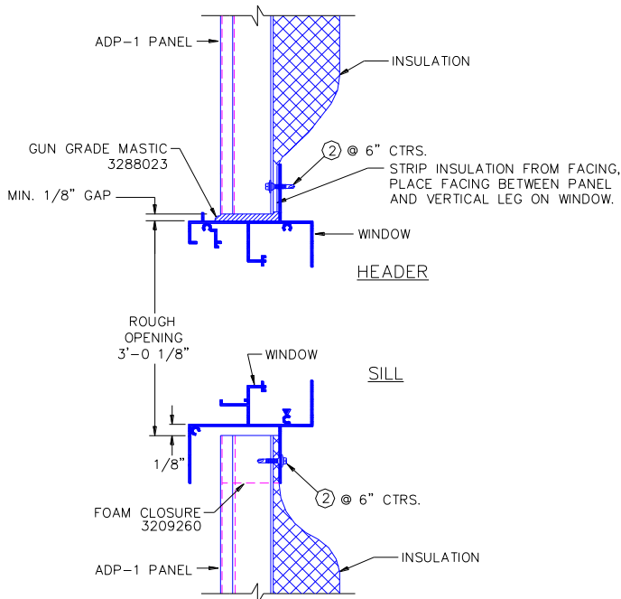
IL. 6.24 SECCIÓN HASTA LA VIGA Y EL ALFÉIZAR
