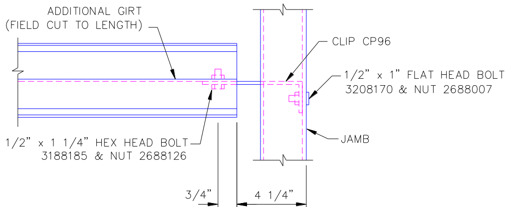
IL. 6.18 FIJACIÓN DE LÍNEAS DE VIGUETA ADICIONALES
