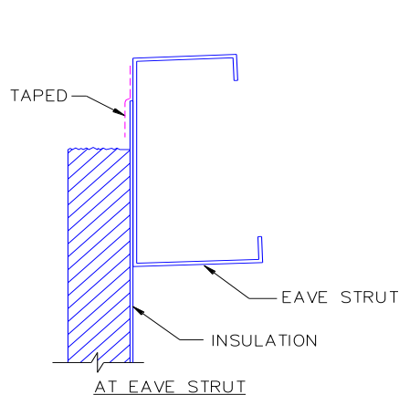
IL. 5.7 AISLAMIENTO ENCINTADO EN LA PARTE SUPERIOR
