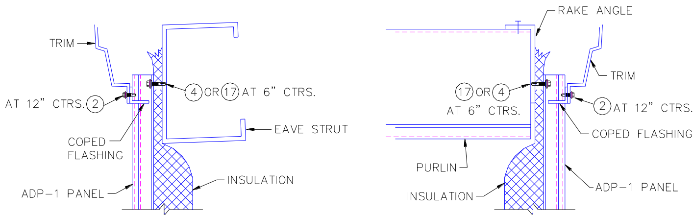
IL. 5.29 MOLDURAS DE PERÍMETRO DE TECHO EN PARTE SUPERIOR DE PANEL DE PARED
