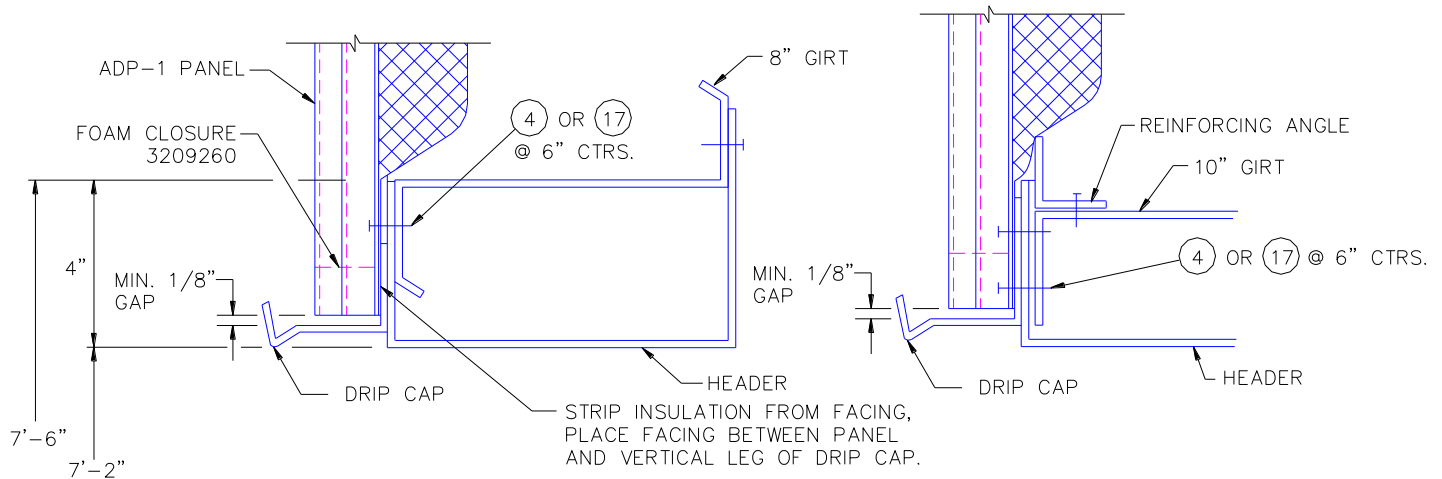
IL. 6.32 PANELES EN VIGA
