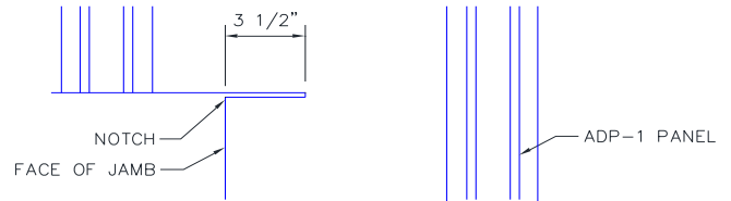
IL. 6.3 CORTE DE PANELES PARA ENCAJE DE CASQUETES DE GOTERÓN
