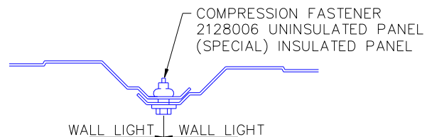
IL. 6.39 SUPERPOSICIÓN LATERAL DE PANELES TRANSLÚCIDOS
