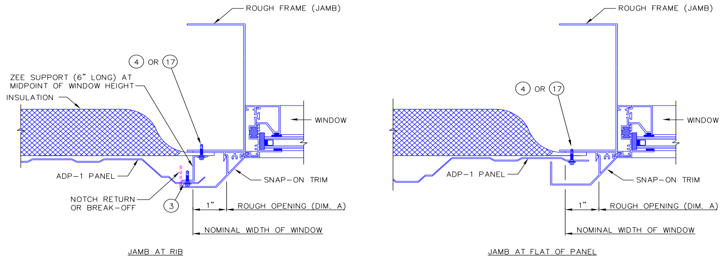
IL. 6.23 SECCIÓN HASTA JAMBA
