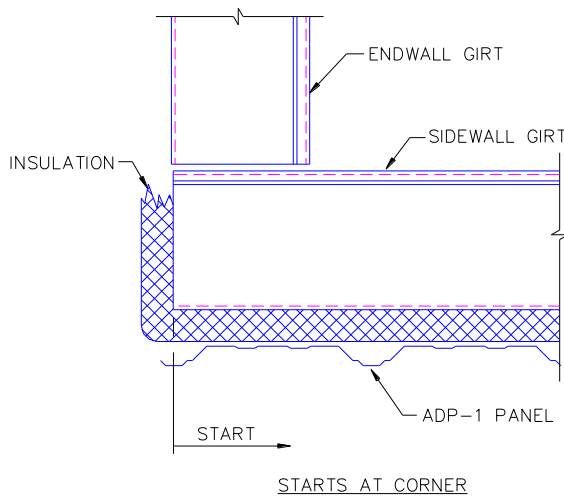
IL. 5.22 COLOCACIÓN DEL PANEL EN LA ESQUINA
