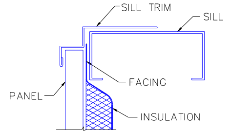
IL. 5.11 EN ALFÉIZAR
