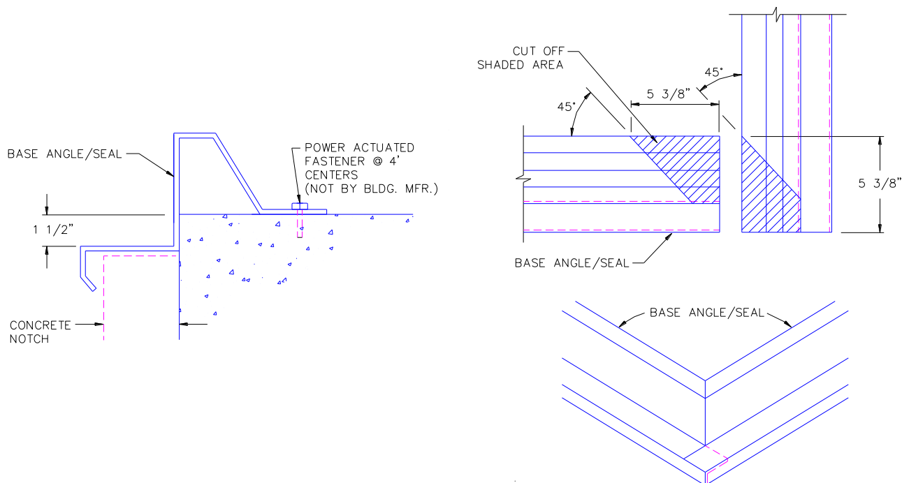
IL. 5.14 SELLO/ANGULAR DE BASE EN LA PARTE INFERIOR DEL PANEL DE PARED
