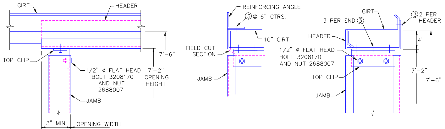
IL. 6.29 CONEXIONES DE VIGA Y JAMBA A VIGUETA
