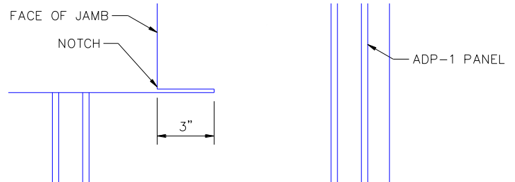
IL. 6.35 CORTE DE PANELES PARA ENCAJE DE MOLDURA DE ALFÉIZAR
