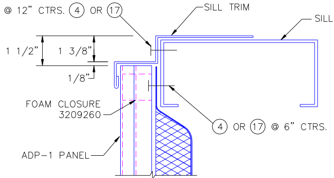
IL. 6.34 PANELES EN ALFÉIZAR
