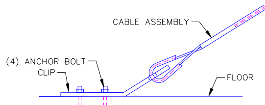
IL. 2.7 ENSAMBLAJE DE GRAPA CONTRA SUELO
