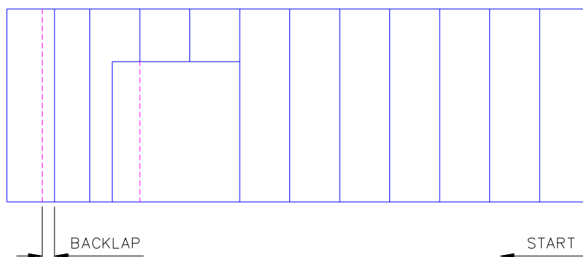
IL. 5.19 PARED LATERAL POSTERIOR (VISTA DESDE AFUERA DE LA ESTRUCTURA)
