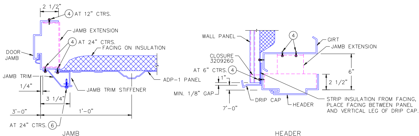
IL. 6.14 SECCIONES EN JAMBAS Y VIGA
