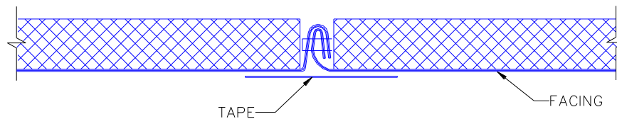
IL. 5.4 JUNTA REFORZADA CON CINTA (OPCIONAL)
