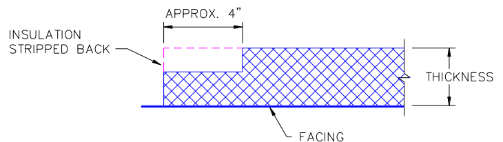
IL. 5.6 EXTRACCIÓN DEL AISLAMIENTO
