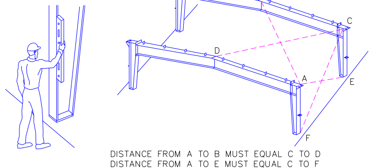
IL. 2.8 NIVELADO Y A ESCUADRA
