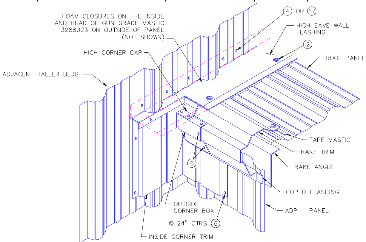
IL. 5.28 ESQUINA INTERIOR DEL ALERO SUPERIOR
