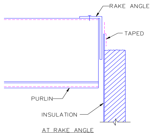
IL. 5.7 AISLAMIENTO ENCINTADO EN LA PARTE SUPERIOR
