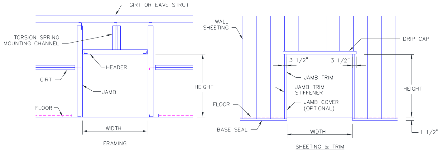
IL. 6.1 ABERTURAS ENMARCADAS PARA PUERTAS BASCULANTES
