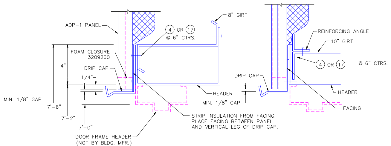
IL. 6.19 PANELES EN VIGA
