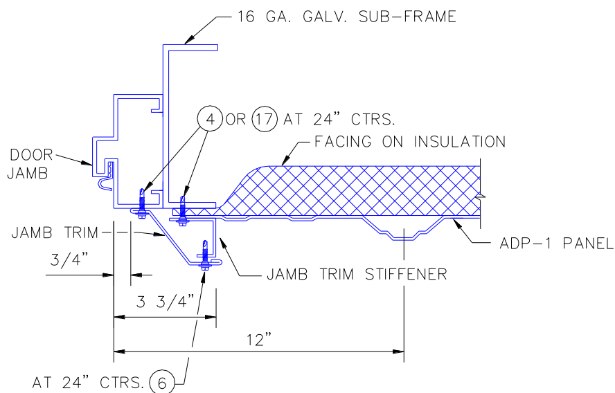
IL. 6.12 SECCIÓN EN JAMBAS
