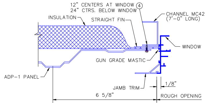
IL. 6.25 SECCIÓN HASTA JAMBA
