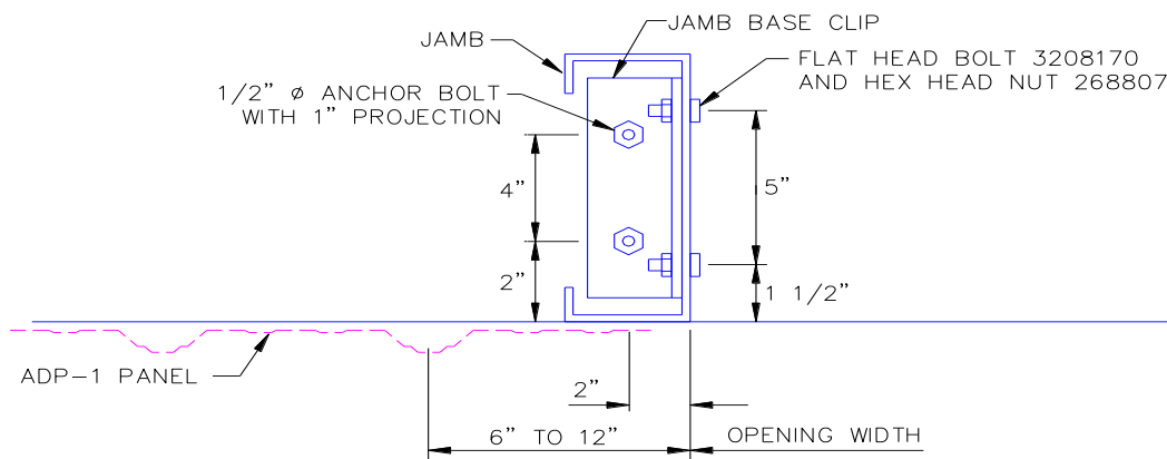
IL. 6.28 DISPOSICIÓN DE JAMBA Y PERNOS DE ANCLAJE EN PUERTA
