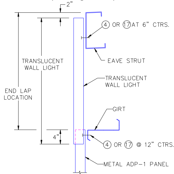
IL. 6.37 LUZ DE PARED TRANSLÚCIDA
