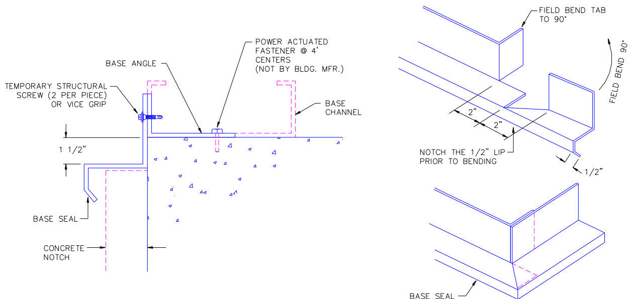
IL. 5.13 SELLO DE BASE EN LA PARTE INFERIOR DEL PANEL DE PARED
