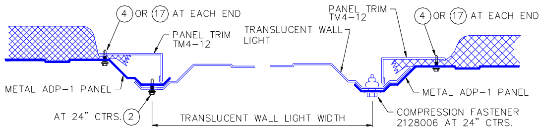
IL. 6.38 SUPERPOSICIÓN LATERAL ENTRE PANEL TRANSLÚCIDO Y PANEL DE METAL
