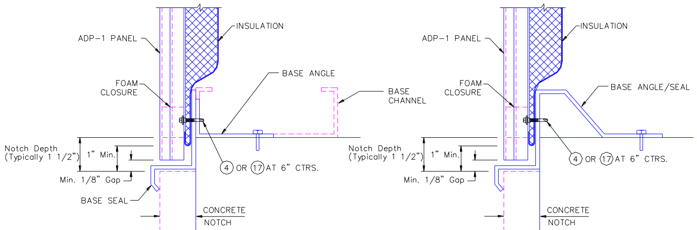
IL. 5.15 CIERRES DE ESPUMA EN LA BASE DE LA PARED
