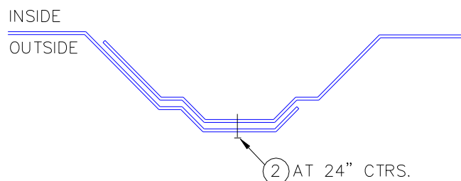
IL. 5.24 SUPERPOSICIÓN LATERAL DE PANEL ADP-1
