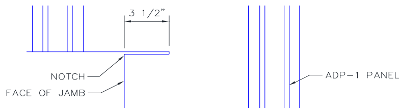
IL. 6.33 CORTE DE PANELES PARA ENCAJE DE CASQUETES DE GOTERÓN
