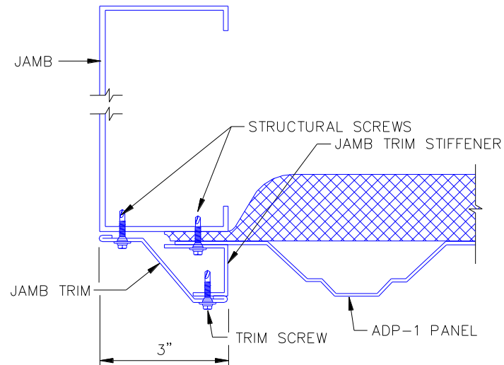
IL. 5.12 EN JAMBAS
