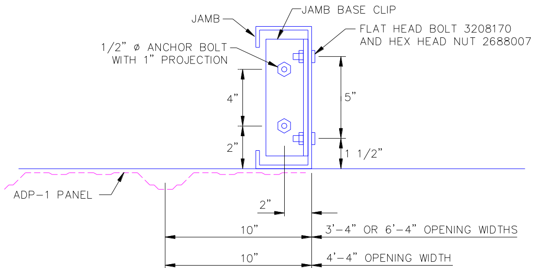
IL. 6.16 DISPOSICIÓN DE JAMBA Y PERNOS DE ANCLAJE EN PUERTA
