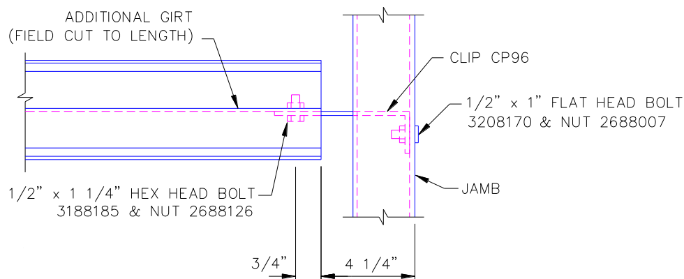
IL. 6.30 FIJACIÓN DE LÍNEAS DE VIGUETA ADICIONALES
