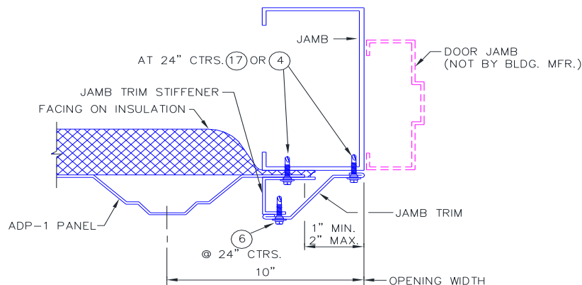
IL. 6.21 MOLDURAS A UN LADO DE LA ABERTURA
